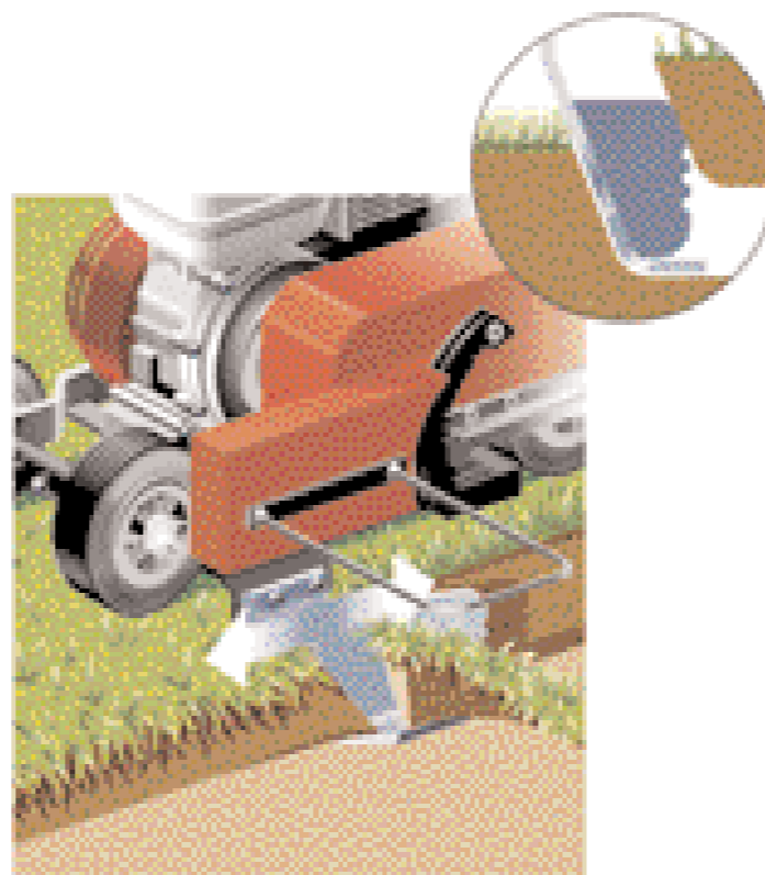
Standardkniv som normalt används på fria kanter. Den finns i olika längder och har en vinge som vänder upp det avskurna materialet och lägger det åt sidan.
