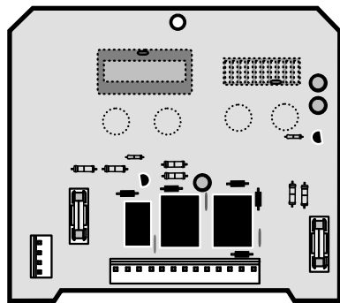
4. P.C.B. PT/NO: 448010100
